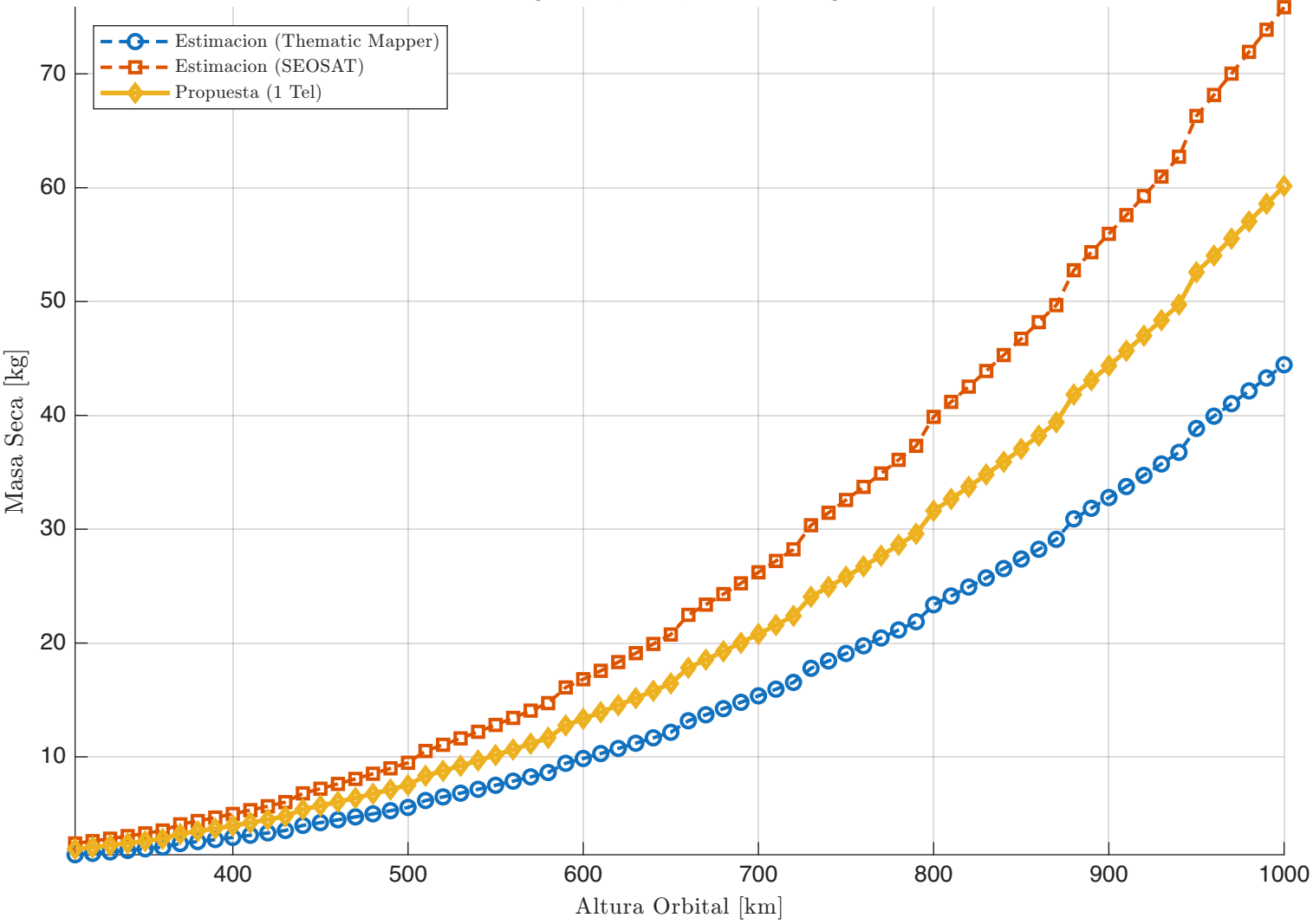
Comparativa de Masa Seca vs. Altura Config: 3 Sat, 1 Tel, Det 3, Cassegrain
